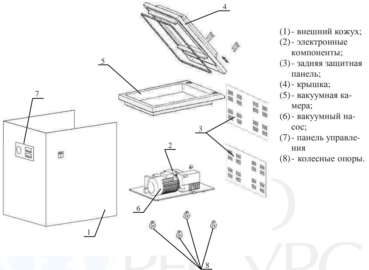
Рисунок 4.4 – Покомпонентный вид справа
