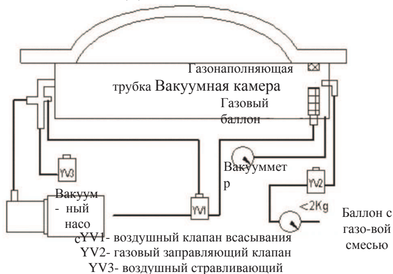
Схема вакуумного упаковщика с системой газации
