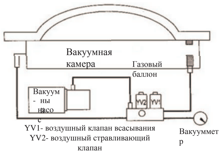
Схема вакуумного упаковщика с производительностью вакуумного насоса более 20 м 3
