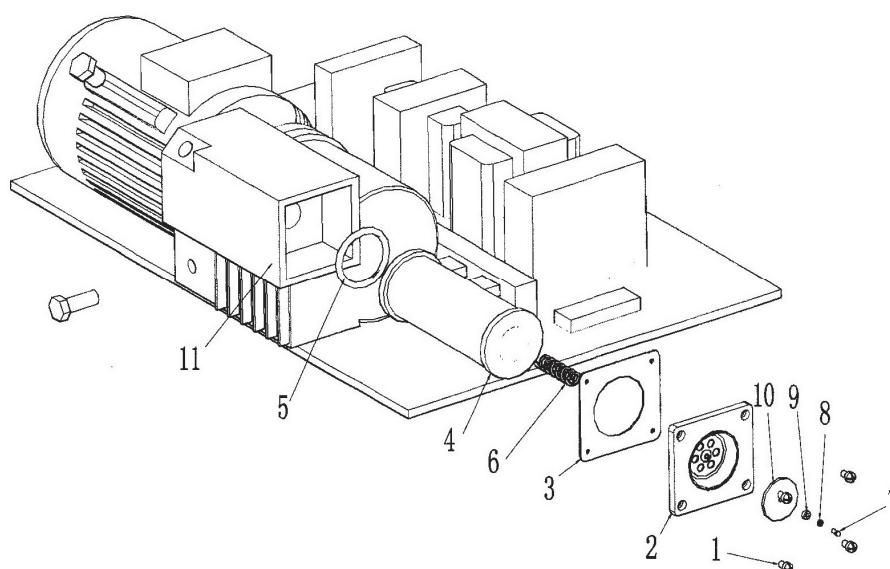
Рисунок 7.3 - Схема элементов вакуумного насоса модели 020
